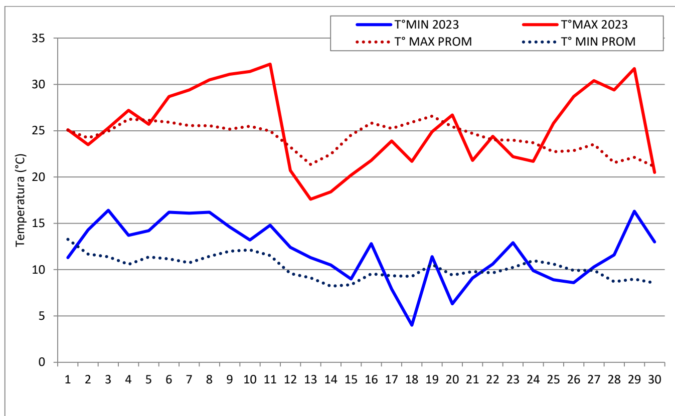
Gráfico 3. Las Temperaturas Máximas y Mínimas Promedios corresponden registros desde el año 2001 hasta el año 2023
