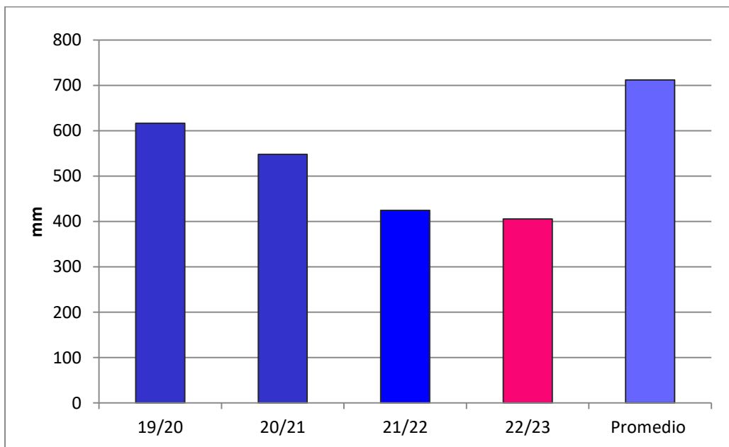
Gráfico 2: Acumulación de precipitaciones durante el periodo julio-abril.
