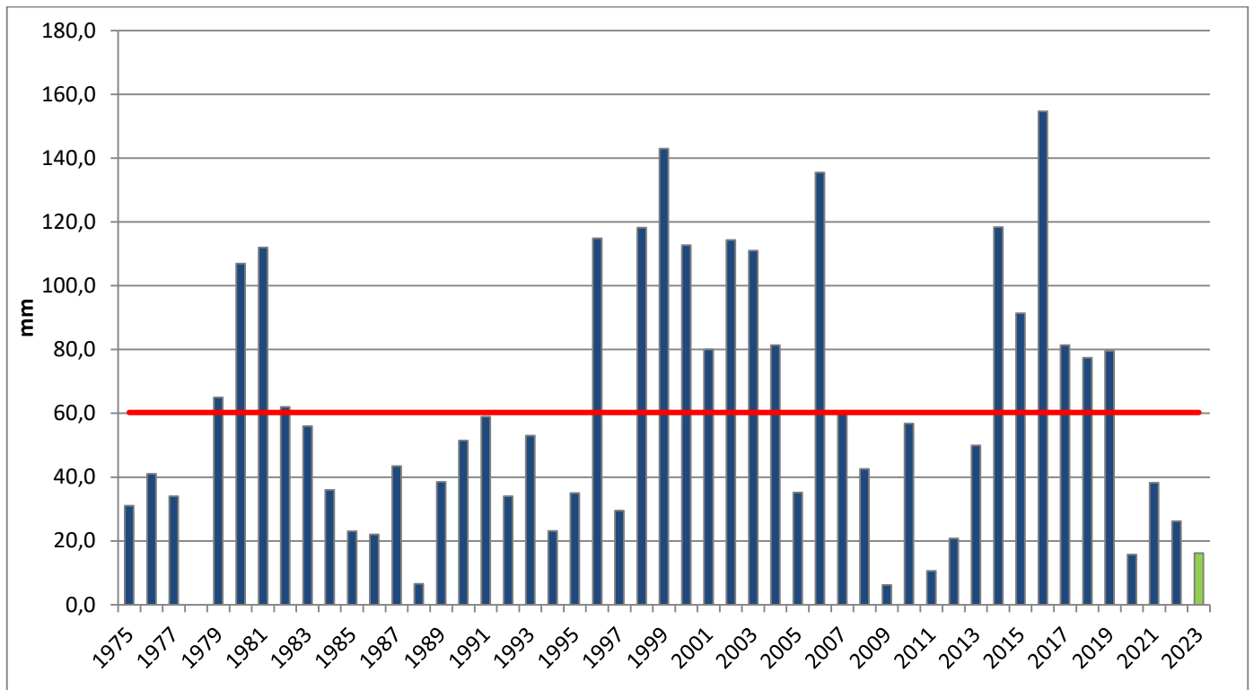
Gráfico 1: Promedio histórico 60,3 mm (línea roja).
