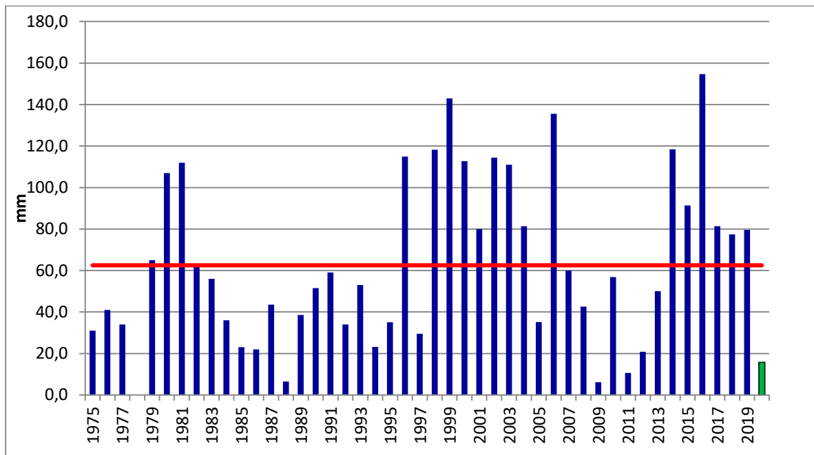
Gráfico 1: Promedio histórico 62.5 mm (línea roja).
