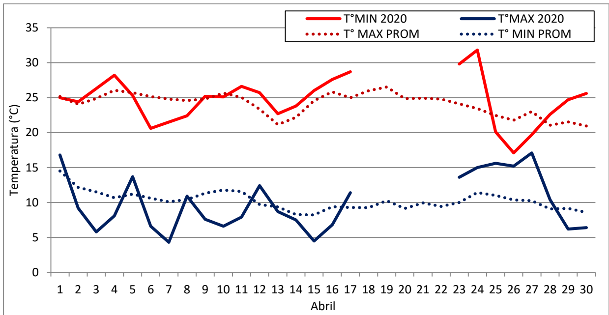
Grafico 3. Las Temperaturas Máximas y Mínimas Promedios corresponden registros desde el año 2001 hasta el año 2020
